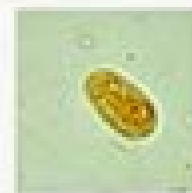
Giardia lamblia
