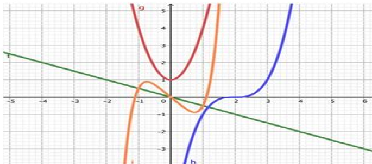
Abbildung 1: Funktionsgraphen
