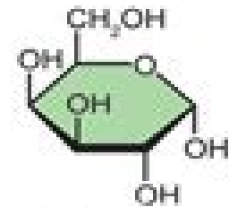
Galactose
