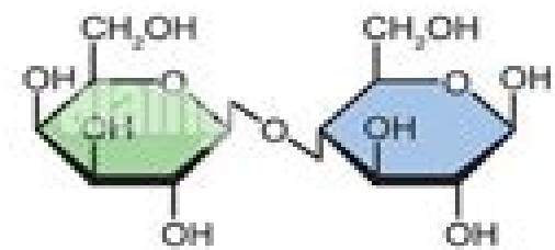
Lactose
