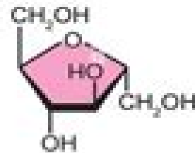
Fructose
