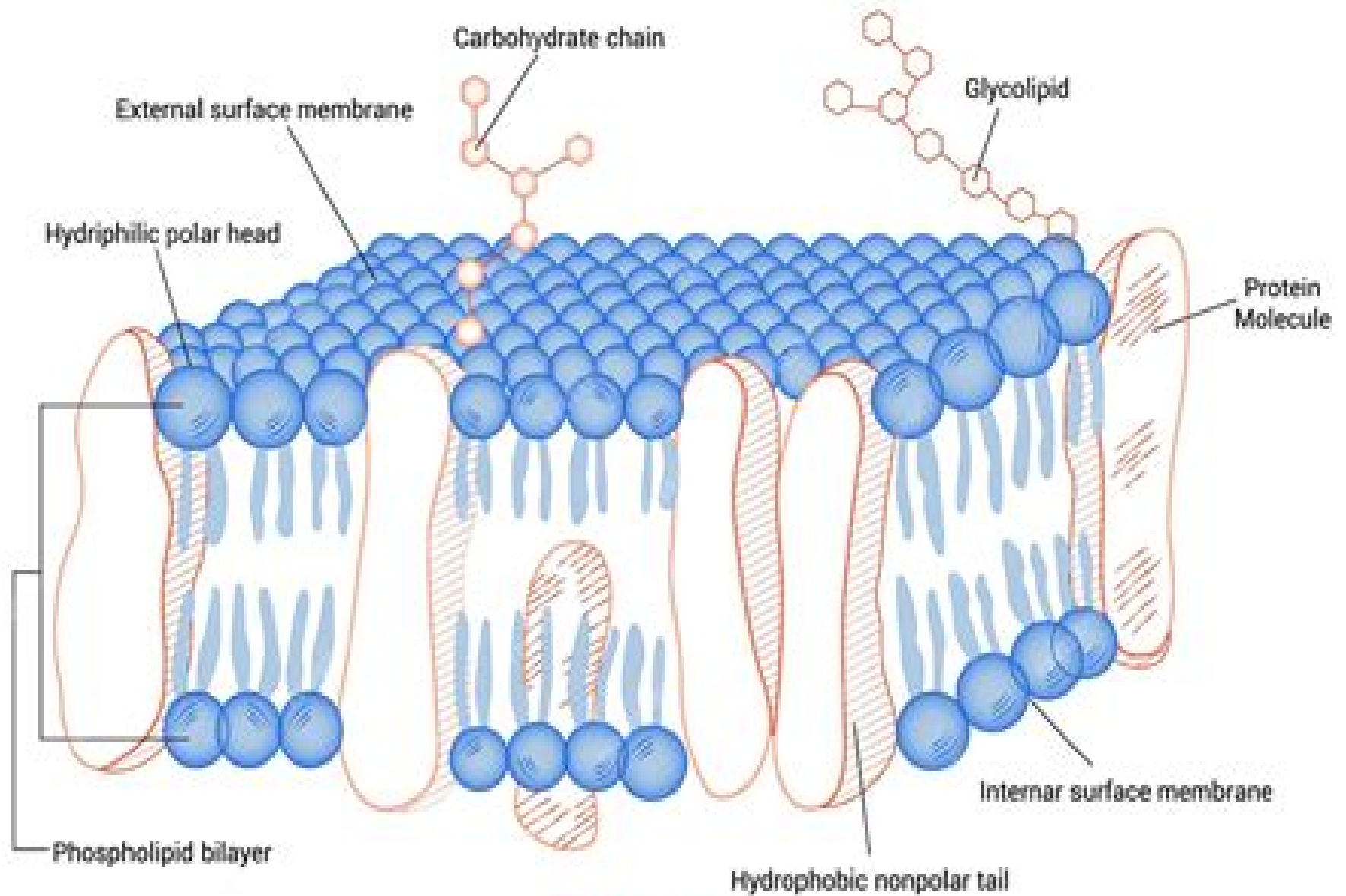
Cell Membrane
