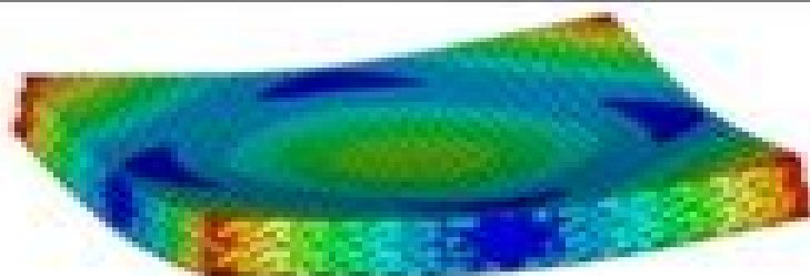
Mode 3: 3389.8 Hz.
