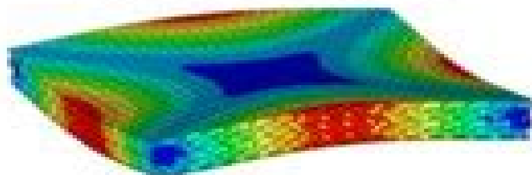
Mode 2: 2781.5 Hz.
