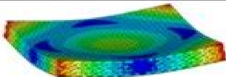
Mode 3: 3389.8 Hz.
