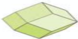
garnet
