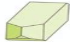
orthoclase
