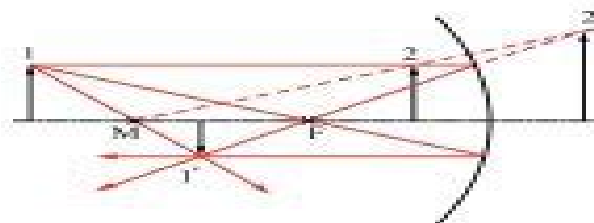
Abb. O.1.0.2 Bildkonstruktion am Hohlspiegel. M Krümmungsmittelpunkt, F Brennpunkt. Die Brennweite ist gleich dem halben Krümmungsradius: f = R/2 .
