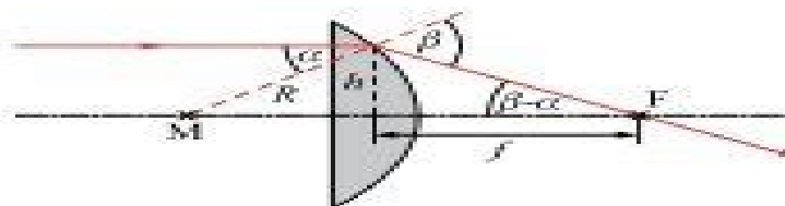
Abb. O.1.0.3 Zur Berechnung der Brennweite einer dünnen Plankonvexlinse
