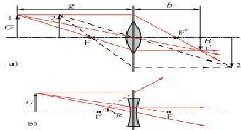
Abb. O.1.0.1 Bildkonstruktion a) bei einer dünnen Sammellinse und b) einer Zerstreuungslinse. G und B bezeichnen Gegenstands- und Bildgröße, g und b Gegenstands- und Bildweite; optische Achse (Strich-Punkt-Linie)
