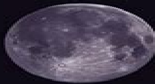
Moon Earth
